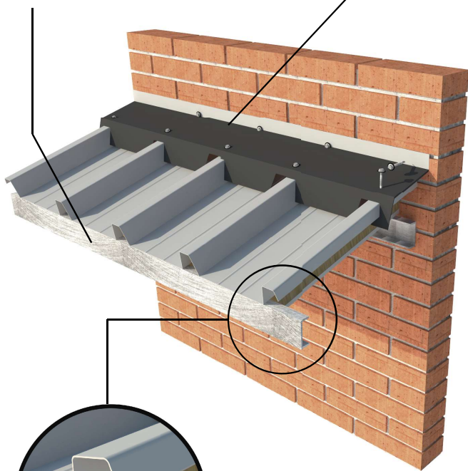
CORREA DE CIERRE
